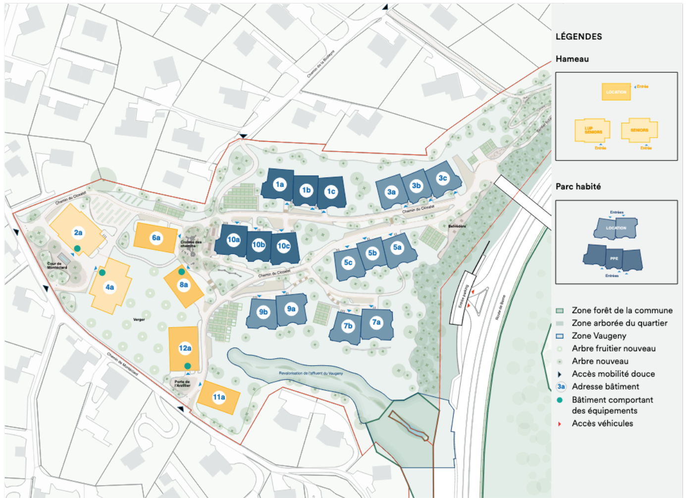
Plan de situation du quartier du Cloalet (RDR ARCHITECTES)
